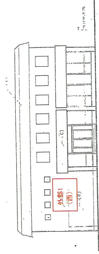
西 面 立面図
