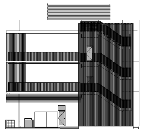
立面図 東
