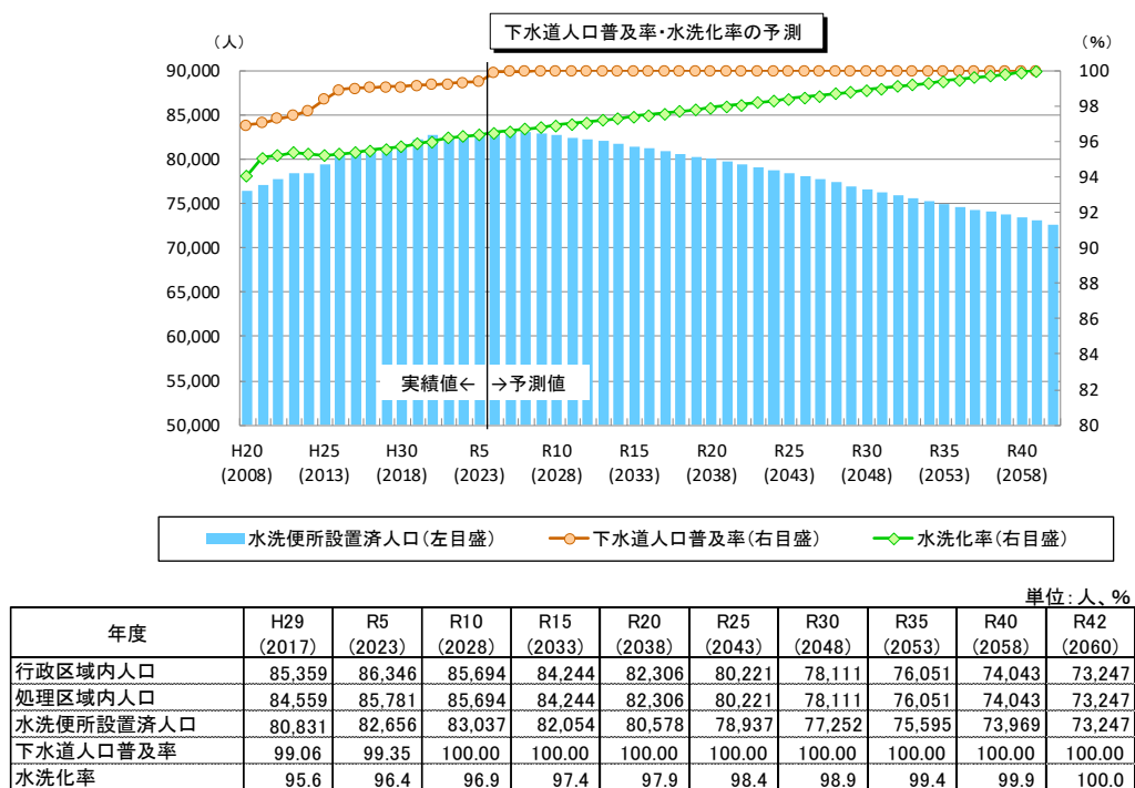
図 4-3 下水道人口普及率、水洗化率の予測結果（見直し）
