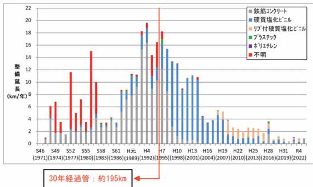
図 2-7 管種別管渠延長（令和 5（2023）年度末現在）
