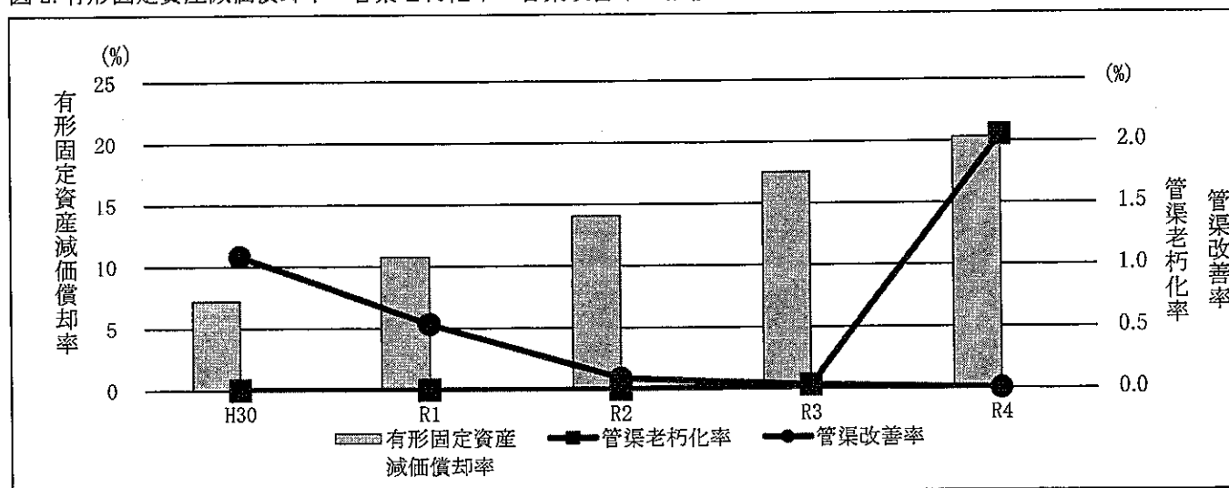
図 2. 有形固定資産減価償却率・管渠老朽化率・管渠改善率の推移
