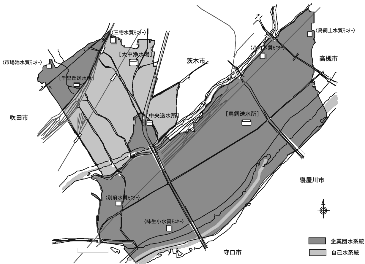
図-1 自己水・受水の水系区域及び浄水場・送水所・水質モニターの位置図
