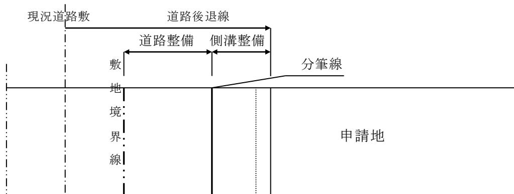
断面図
