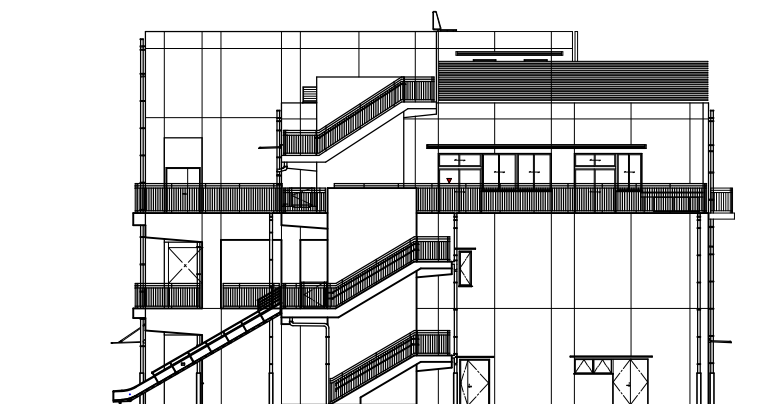
南東側立面图
