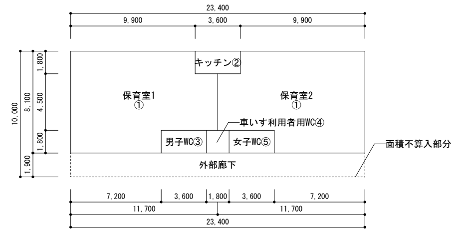
1階
